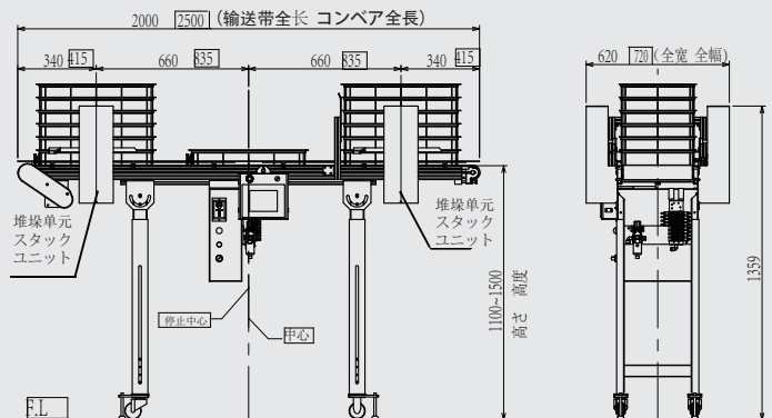
*外形尺寸图为A-40基本尺寸。□内表示A-70的尺寸。 図面はA-40です。□は、A-70の寸法を示します。 This drawing is for A-40. Figures in □ show the sizes of A-70 II.
